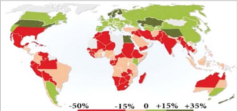
تصویر ۲: مدل تأثیر تغییرات اقلیم بر تولیدات گیاهی تا سال ۲۰۸۰ میلادی
