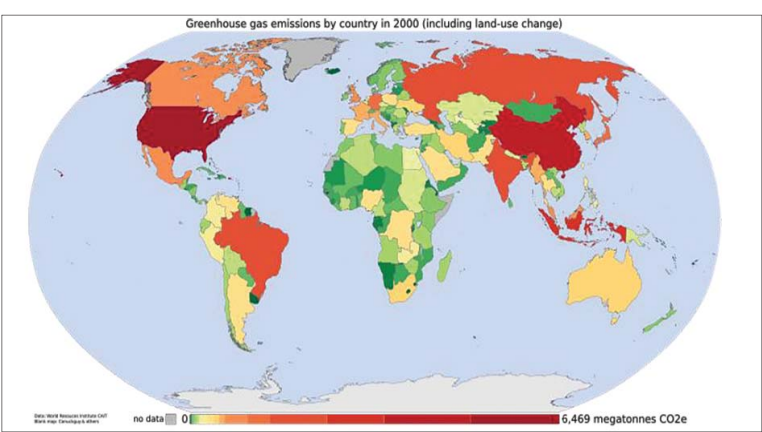
تصویر ۱: میزان کاهش کشورها در تولید گازهای گلخانه‌ای (از گزارش‌های سیاست‌گذار IPCC)
